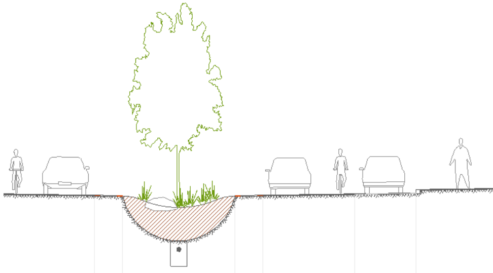
Mynd 9. Dæmi um jarðvegssú í miðeyju Kjarnagötu. -
