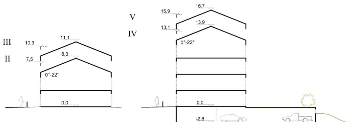
Mynd 13. Hæðir fjölbýlishúsa F II, F III, F IV og F V. Dæmi um bílageymslu.
